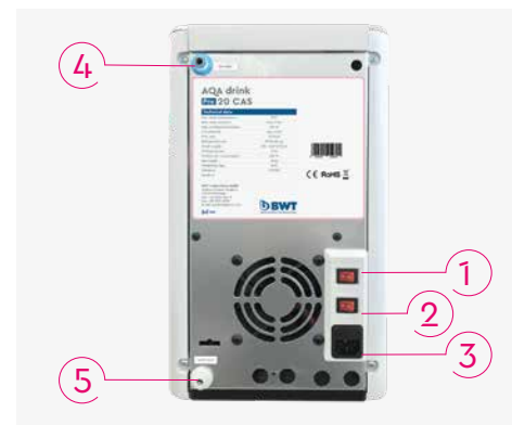
Fig. 3: face arrière de l'AQA drink Pro 20 CAS
